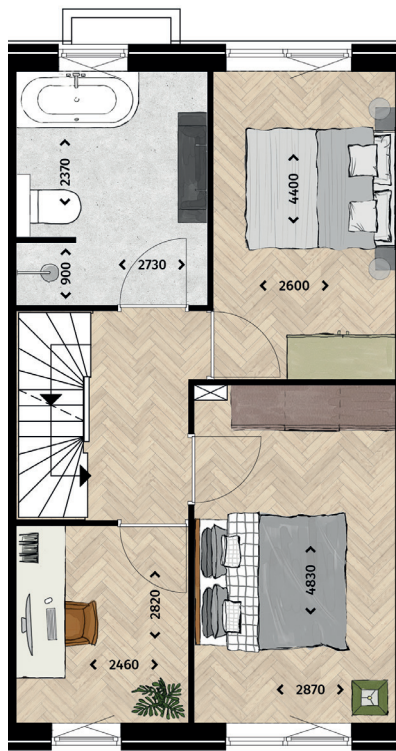
EERSTE VERDIEPING
